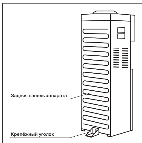
Рис. 2. Фиксация аппарата
