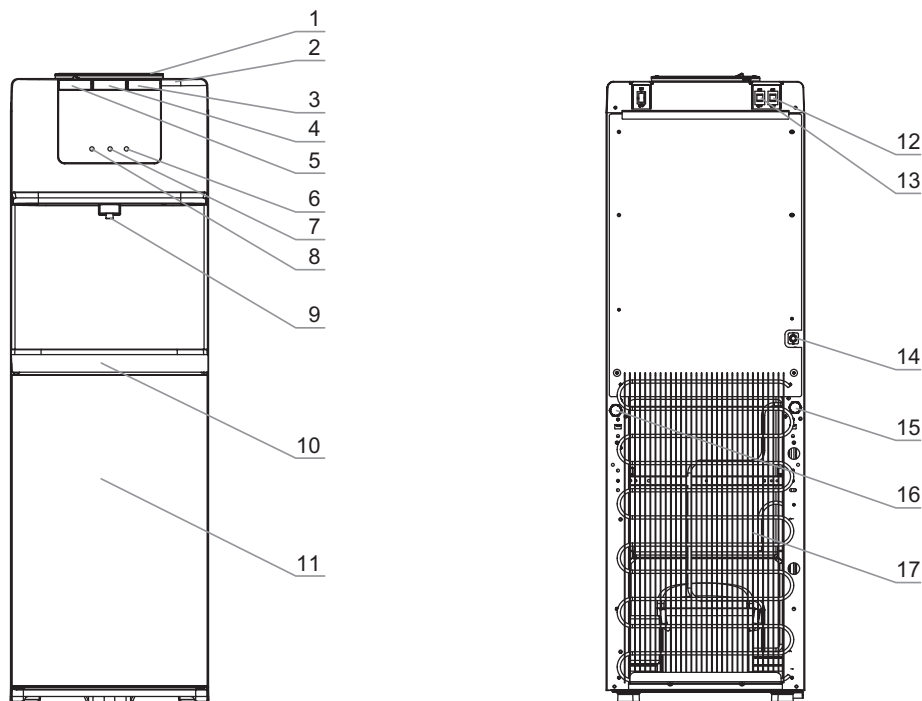
Мал. 1. Схема апарату V8020C
